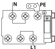
Fig. 2 - Etiqueta de esquema de conexión
