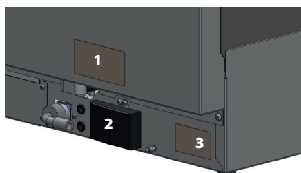
III. 3 – 1. Étiquette du schéma de connexion, 2. Boîte à bornes, 3. Plaque d'identification
