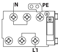
Obr. 2 - Štítek se schématem připojení
