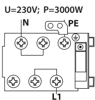
III. 2 - Étiquette du schéma de connexion
