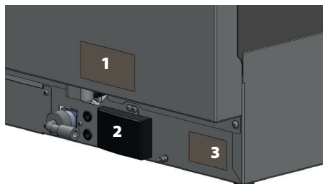
Fig. 3 – 1. Etiqueta del esquema de conexión; 2. Caja de conexiones; 3. Placa de características
